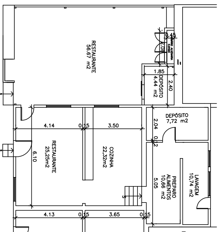
PLANTA BAIXA RESTAURANTE EEN
